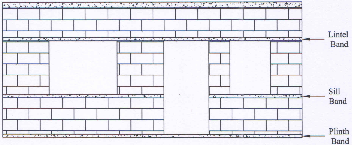
ELEVATION
